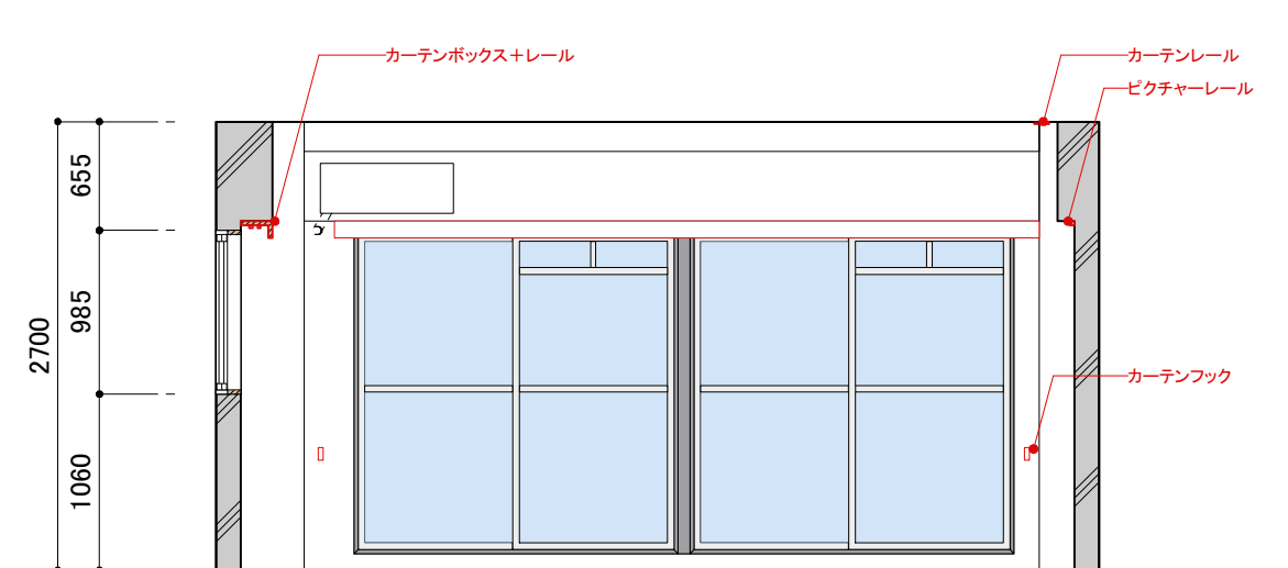
D 展開図
