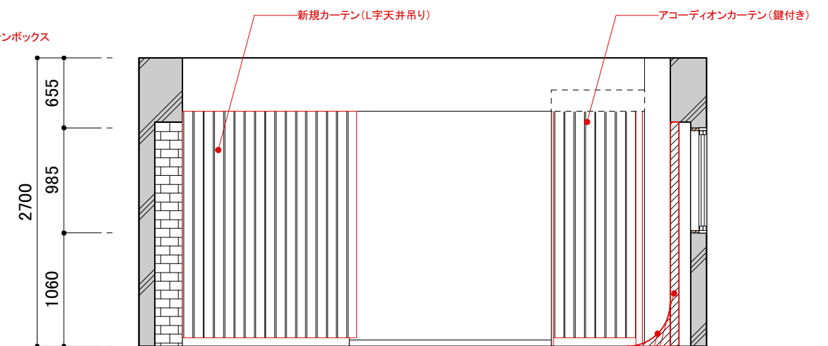
E 展開図
