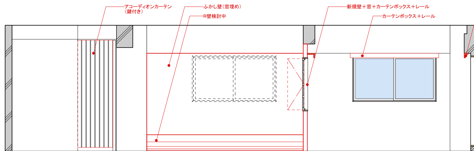
C 展開図
