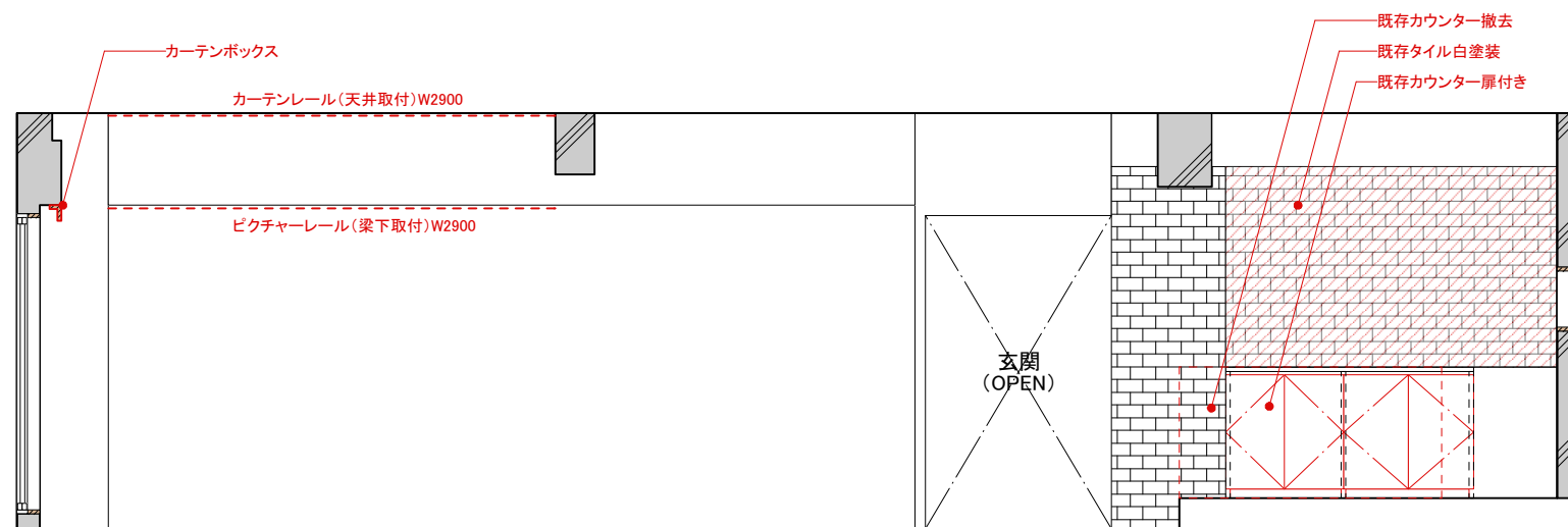
A 展開図
